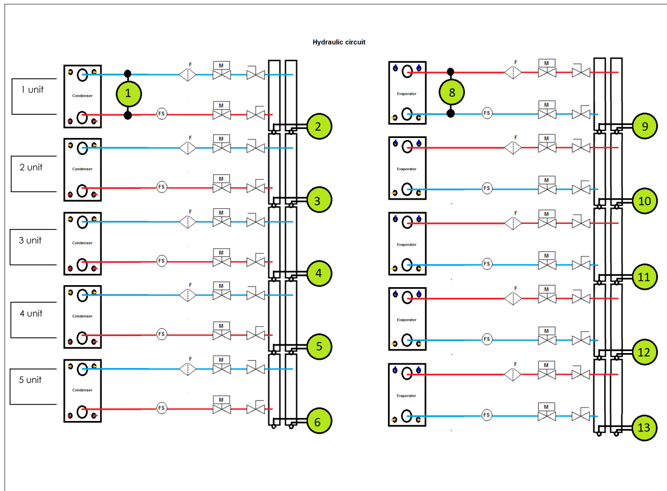
Figura 8. Configuración de circuito hidráulico.
