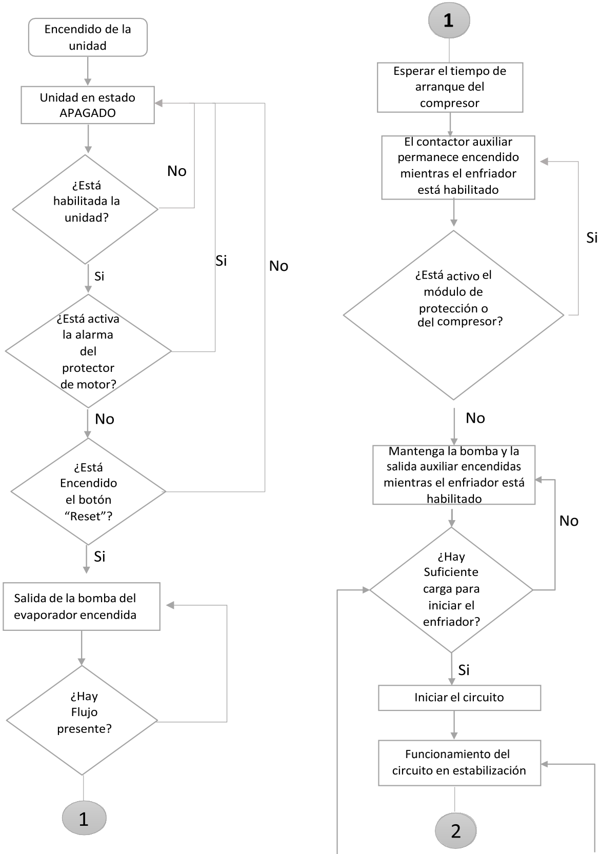
Figura 21. Secuencia de funcionamiento de la unidad.
