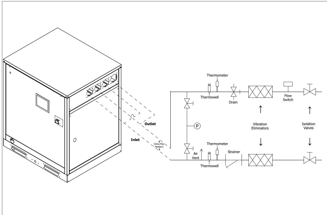
Figura 3. Tuberías típicas de un evaporador de placas soldadas, serie CLIM LC Tandem
