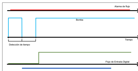
Figura 16. Ejemplo del ciclo de la puesta en marcha de la bomba, donde el flujo se detectó en segundo intento
