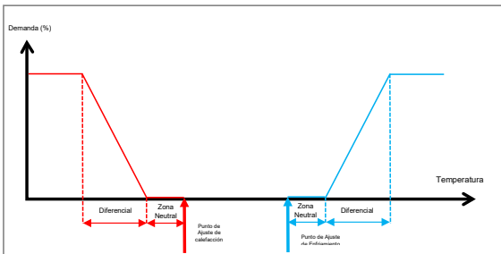
Figura 18. Ejemplo del ciclo de control proporcional, para casos de demanda total o demanda para la unidad "Madre"
