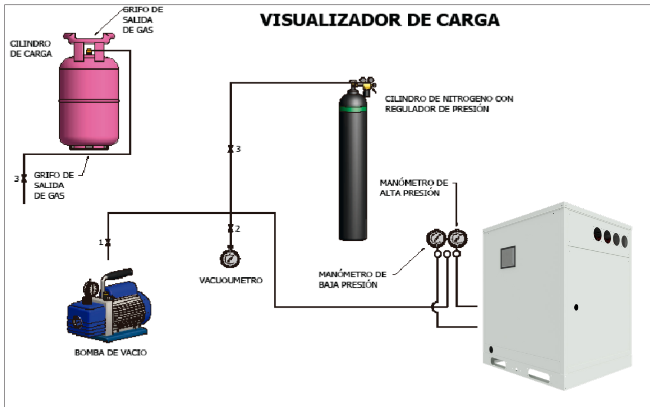
Figura 7. Diagrama para obtener el vacío y carga de refrigerante.
