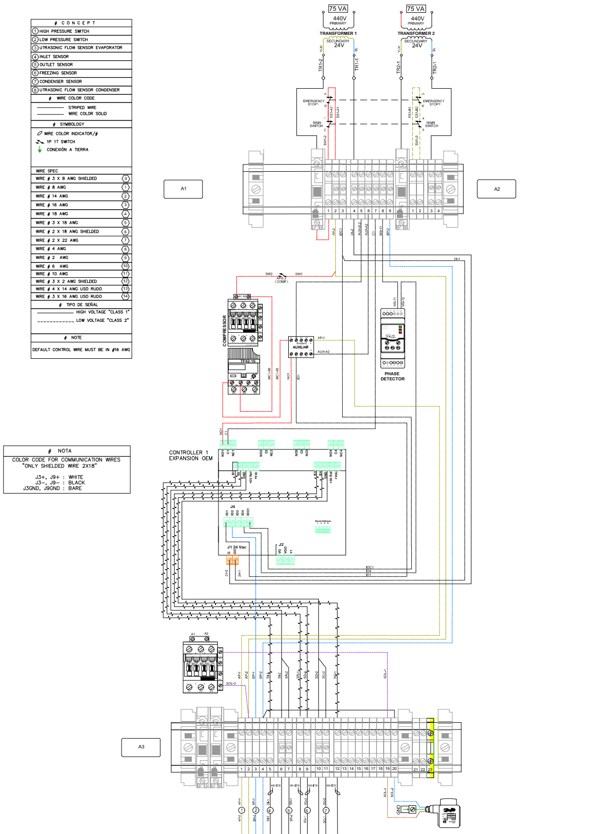
Figura 10. Diagrama de cableado de campo típico de la unidad CLIM LC 7.5 TR hijo 440V (conexión multi-punto con todas las opciones mostradas)
