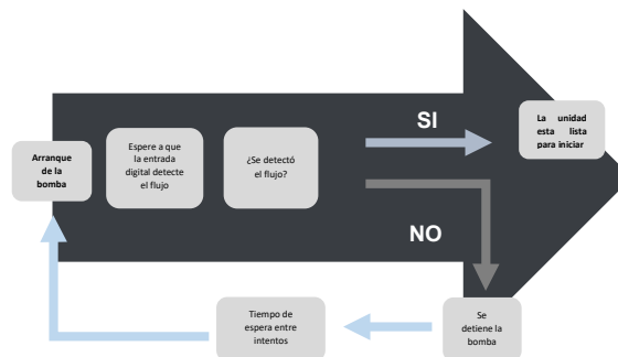
Figura 15. Diagrama de Flujo del control del arranque de las bombas (aplica para cualquier unidad)
