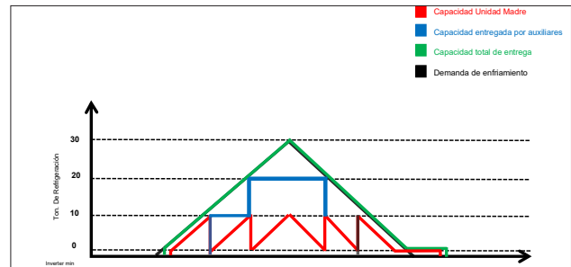
Figura 20. Ejemplo de capacidad entregada de acuerdo a la demanda, para una unidad "Madre" y 2 unidades "Hijos" de 10TR de enfriamiento cada una
