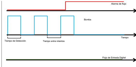
Figura 17. Ejemplo del ciclo de la puesta en marcha de la bomba donde el flujo no ha sido detectado, después de 3 intentos la alarma de flujo ha sido activada
